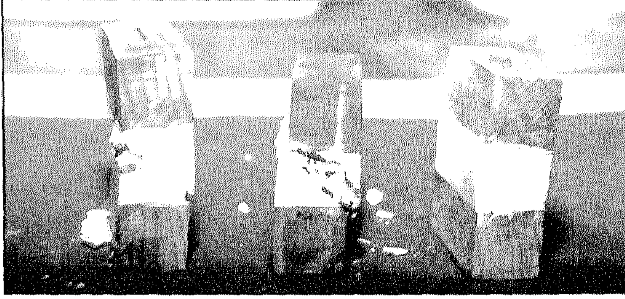
صورة رقم (١٥٦- أ ب ج د هـ و) توضح مدى الاختلاف في ميكانيكية انهيار عينات المعاجين المألثة المختارة المثبتة بين ساقين من خشب صلب أثناء اختبار قياس قوى الضغط حيث:
